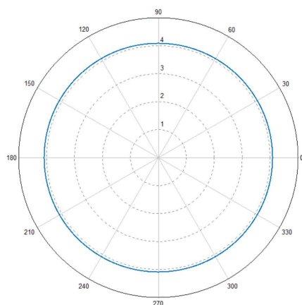
水平方向图
