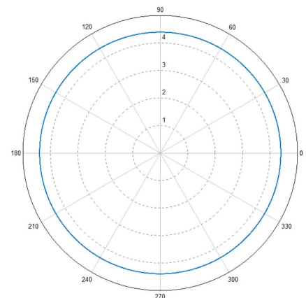
水平方向图
