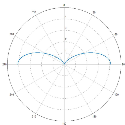
垂直方向图
