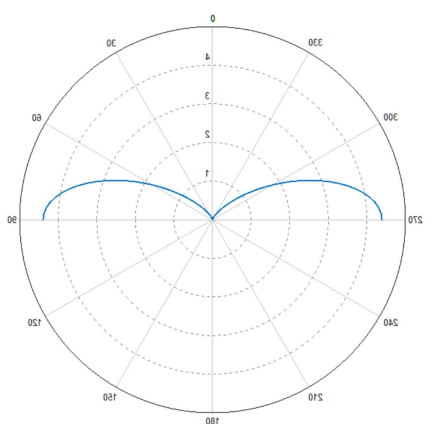
垂直方向图
